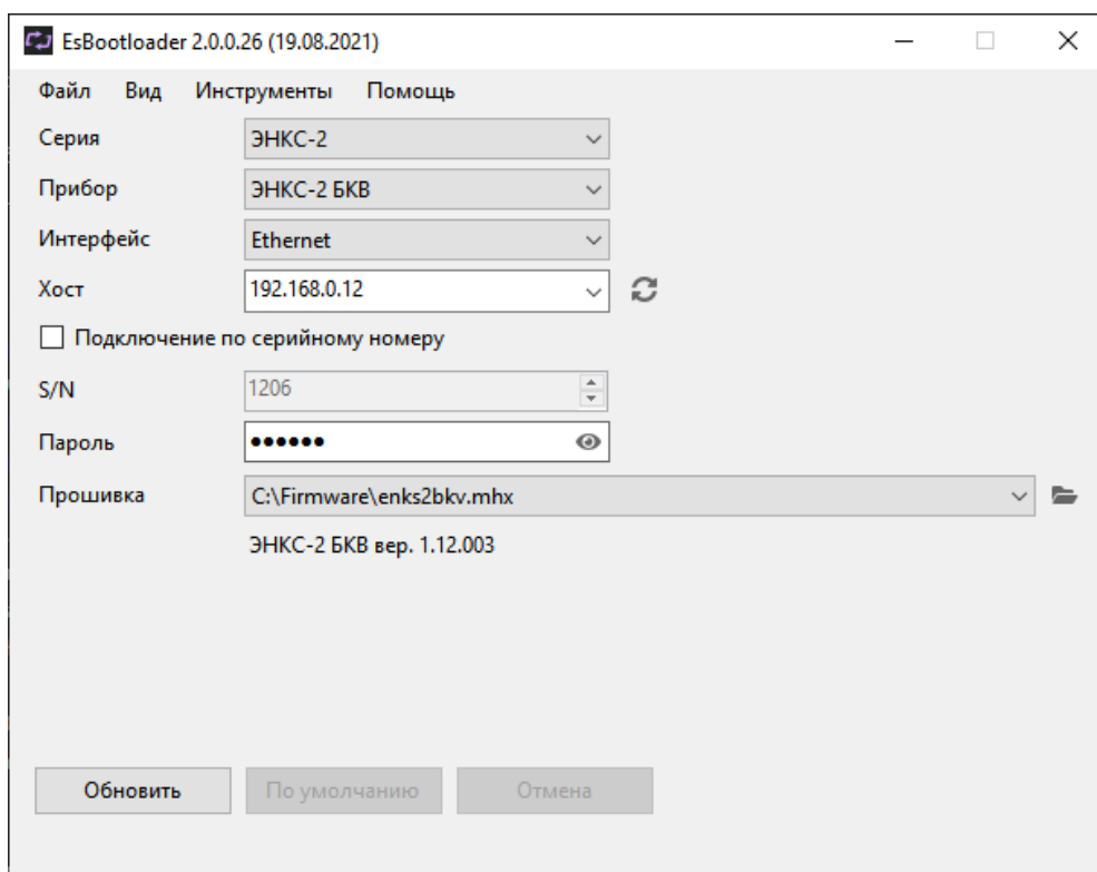
Рисунок 6.1. Интерфейс ПО «ESBootloader»
