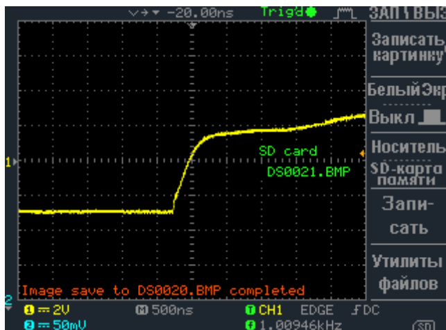
Рисунок 5.4. Линия, согласованная 120 Ом.
