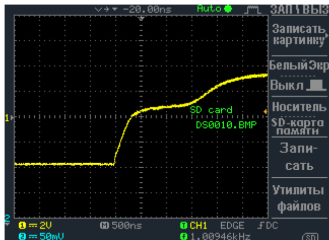
Рисунок 5.2. Линия с «оттяжками» 1 кОм.
