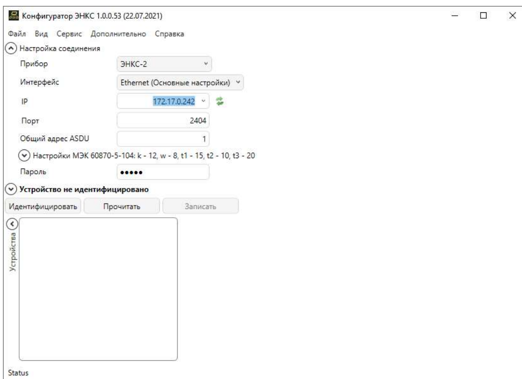
Рисунок 6.6. Стартовое окно конфигуратора
