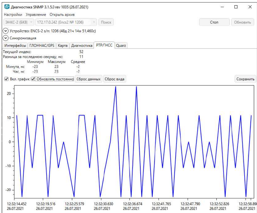
Рисунок 3.1. Статистика разницы часов между PTP и ГЛОНАСС/GPS
