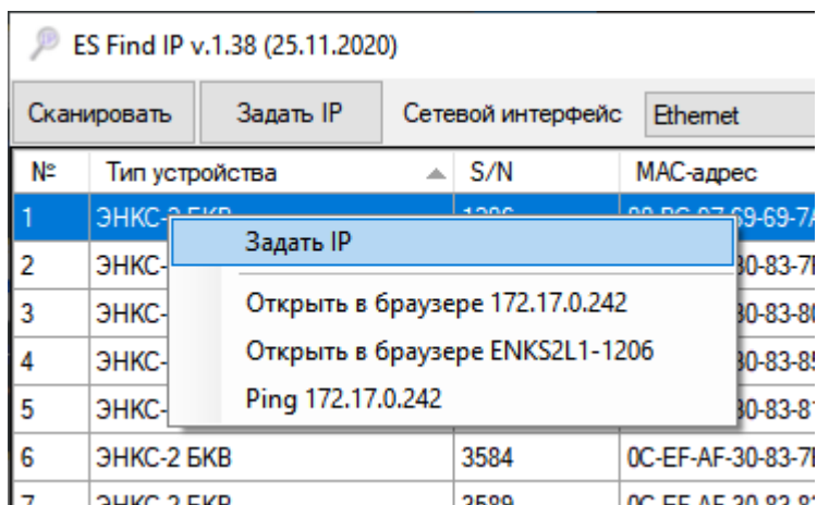
Рисунок 6.3. Окно программы «ES Find IP»
