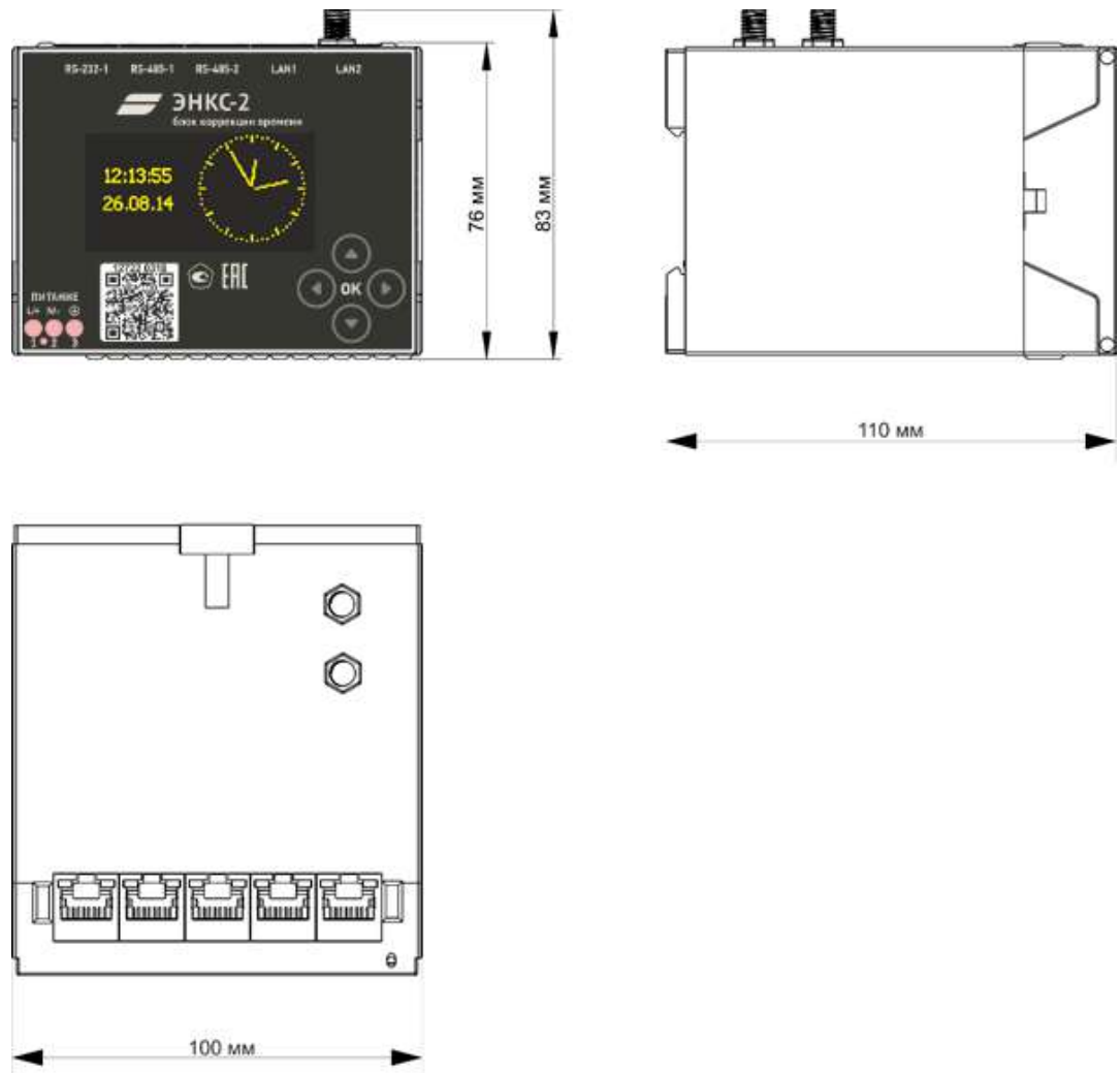
Рисунок 1.3. Габаритные размеры БКВ ЭНКС-2
