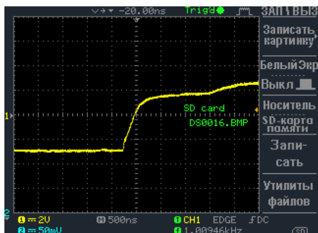
Рисунок 5.3. Линия, согласованная 1 кОм.
